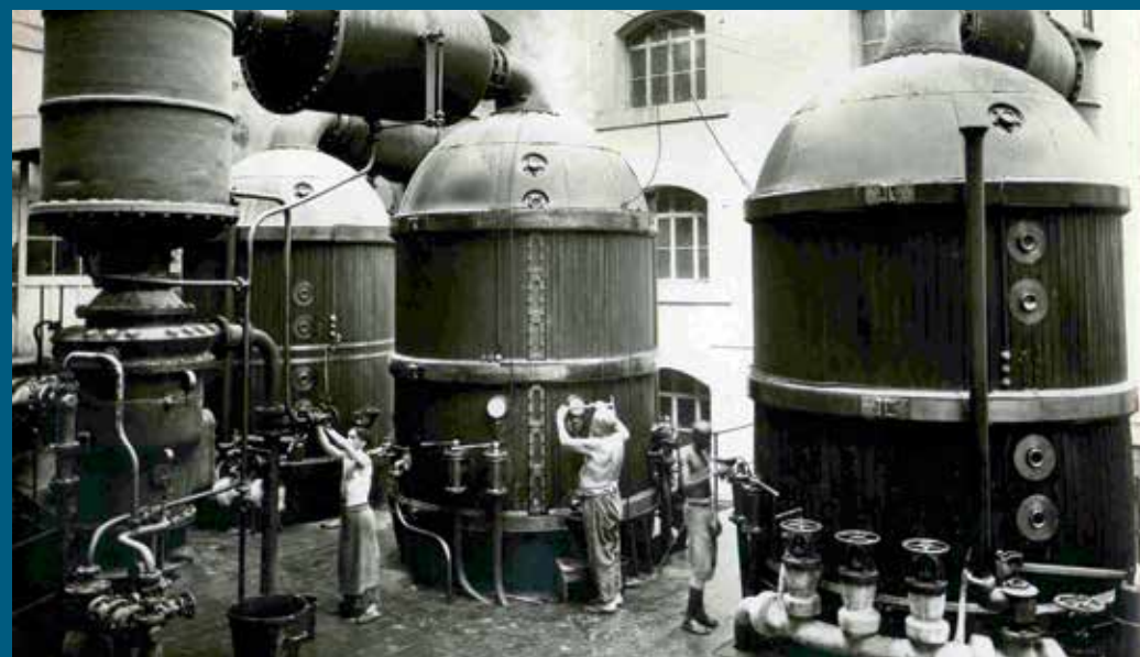
Raffinerie de sucre Saint-Charles appartenant à Saint-Louis : chaudière à cuire, photographie de Mathieu, 1915, 122 Fi 1 © Conseil Général 13 – Archives Départementales.
